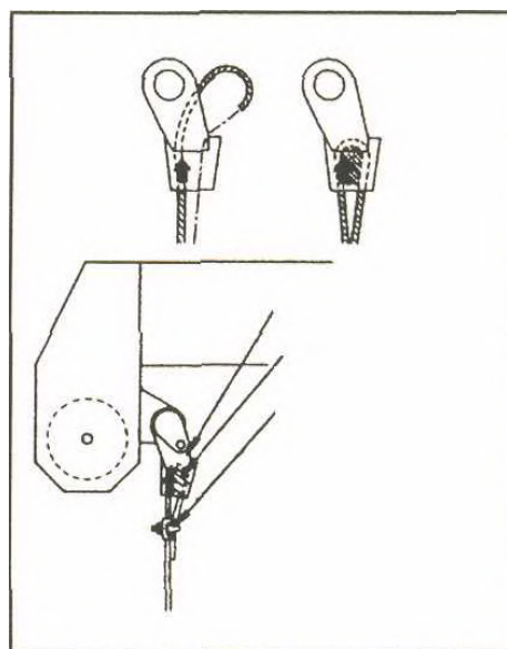
Обжимка каната
