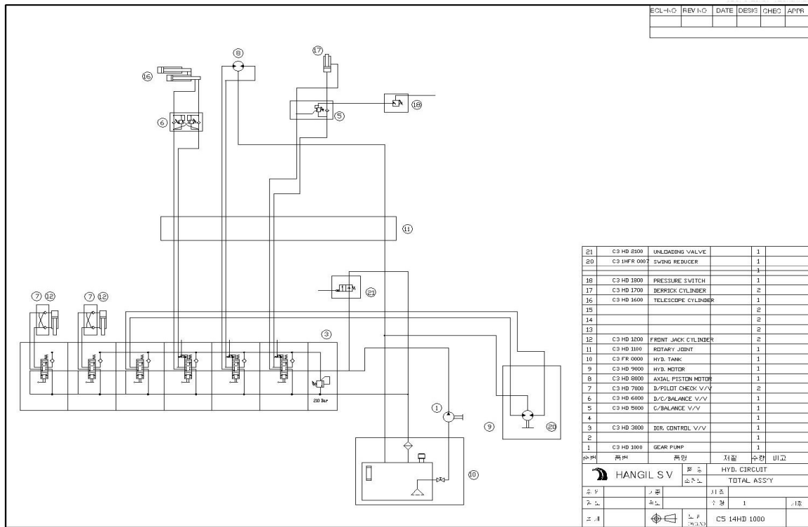
Рис. 5 КМУ модели HGC514
