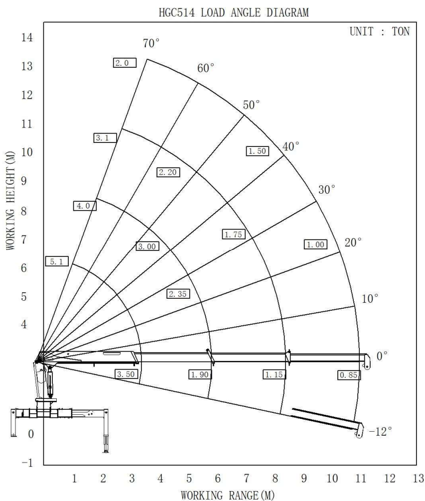
Рис. 2 Диаграмма высотных характеристик КМУ модели HGC514
